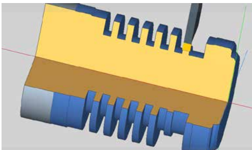
Tronzado con peine: avances de un 30 % a un 50 % mayores mediante parámetros de mecanizado óptimos.
