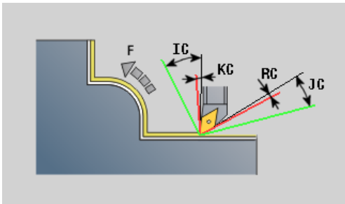
Acabado simultáneo: torner siempre con el ángulo de incidencia óptimo.
